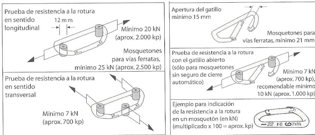
Figure 2. Carabiner break test (Schubert and Stückl, 2007, p.85)
