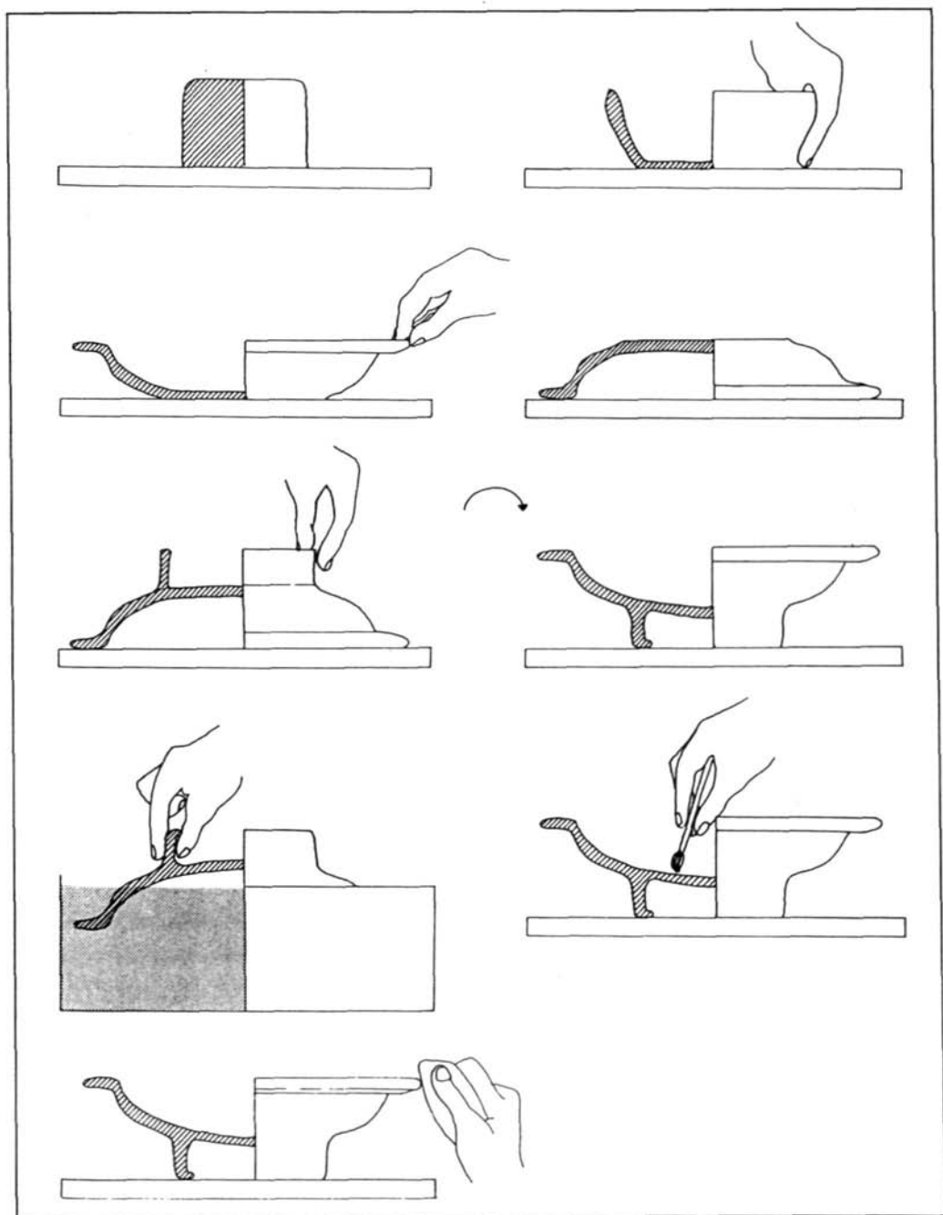
Figura 1. Proceso de fabricación de los platos de Gerasa
