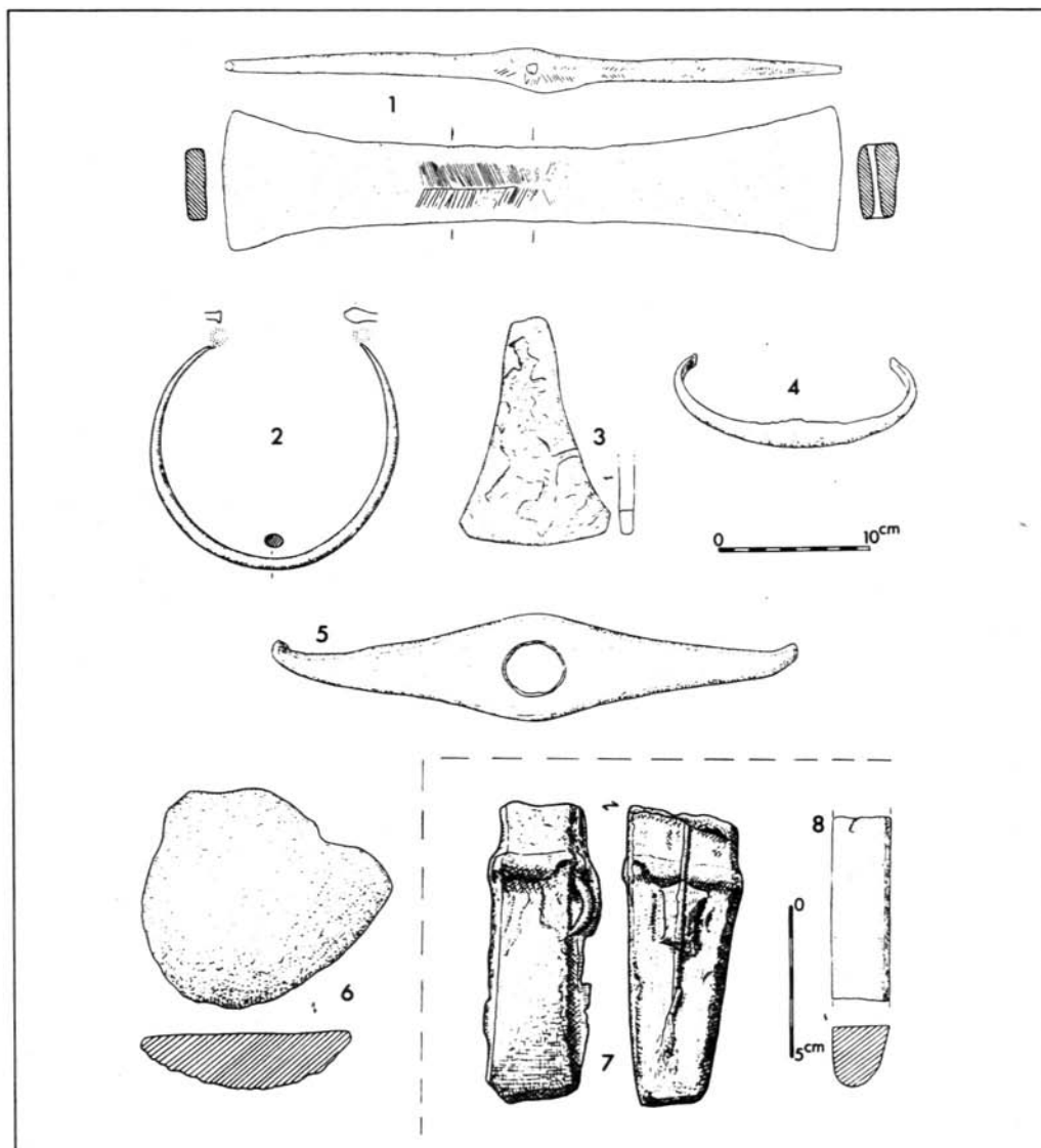
Figura 1. Diferentes tipos de lingotes durante la Edad del Bronce. 1. Lingote bípenné de cobre, 2. Lingote-torque, 3. Lingote en forma de hacha plana, 4. Lingote-barra, 5. Lingote "saumon" de bronce, 6. Lingote plano-convexo de cobre, 7. Lingote de plomo en forma de hacha, 8. Barra de bronce. (J. Briard, 1976, fig. 1, 239)
