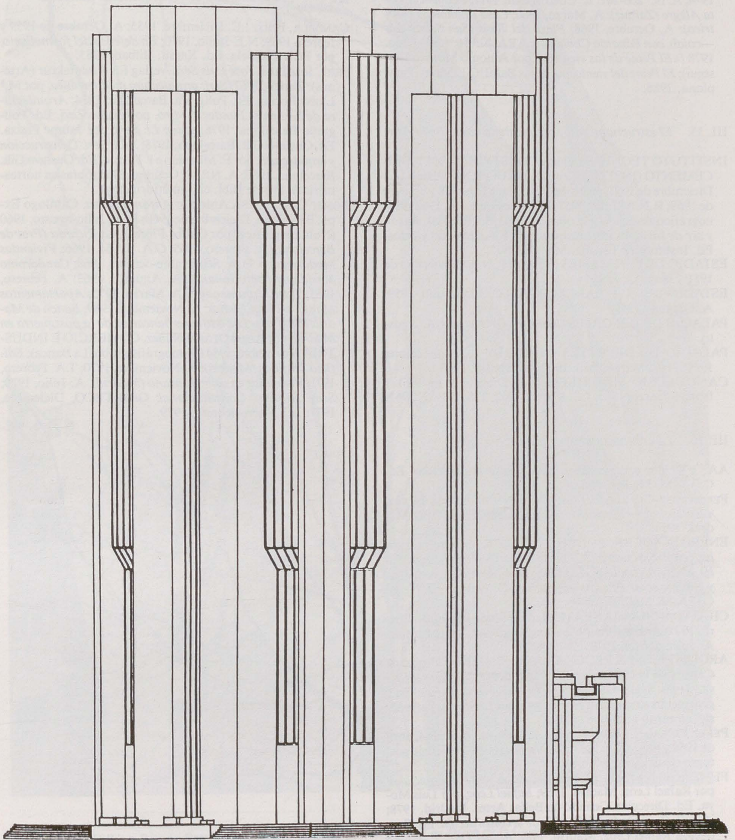
Antonio Fernández Alba: Anteproyecto para Banco de Bilbao en AZCA, 1971, Madrid. Fernández Alba había practicado también durante esos años sesenta la arquitectura organicista en general y próxima a Aalto en particular, pero en la década siguiente orienta su obra hacia un orden mayor e «institucional», al margen de las tipologías y de los materiales corrientes, proceso en el que no se halla ausente la referencia a Kahn. Esta obra evita ser oficina-paisaje en espacio interior, al tiempo que sus ordenados volúmenes positivos in crescendo valoran escultóricamente los espacios negativos.
