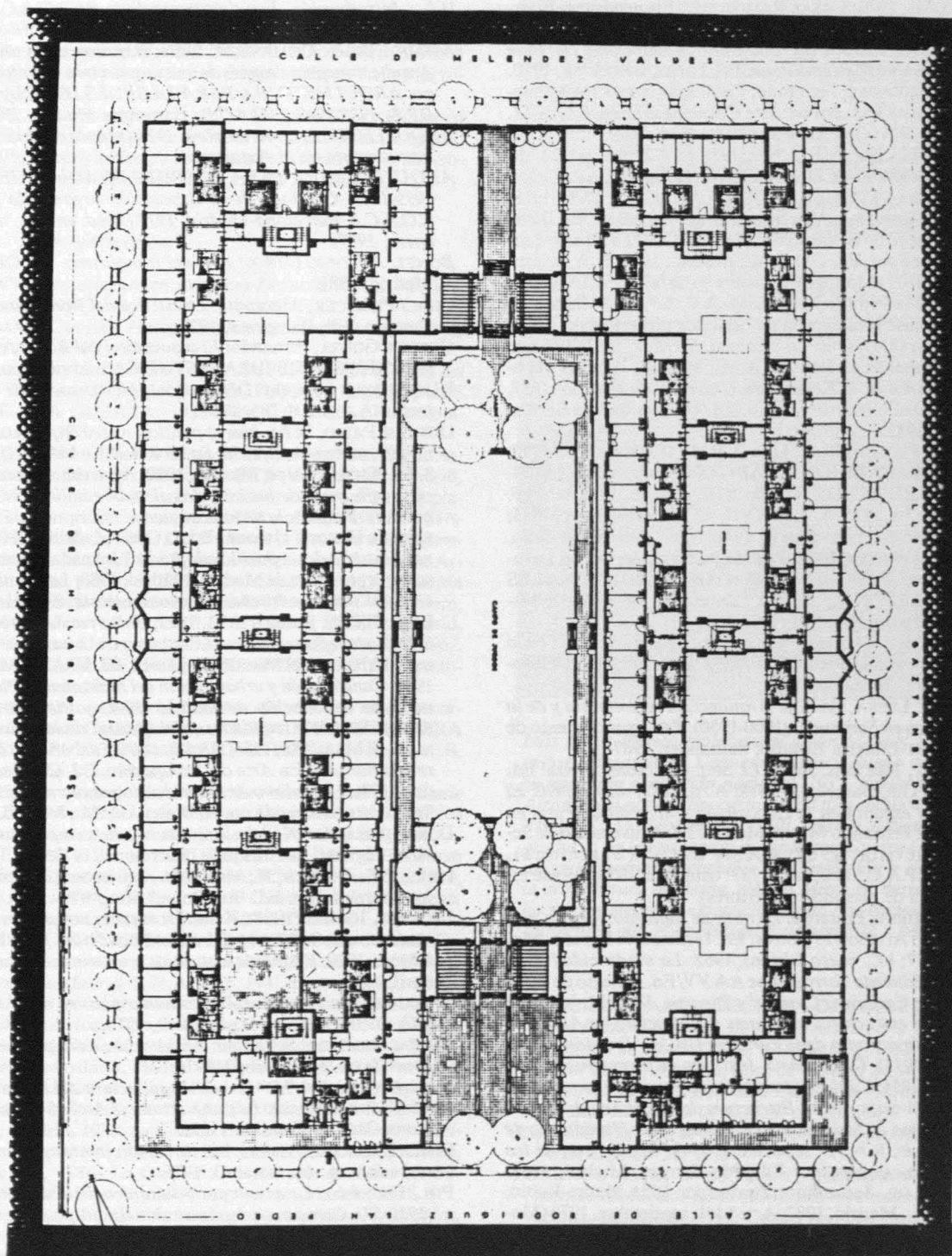
Secundino Zuazo y Miguel Fleischer: Casa de las Flores, 1930-32, Madrid. Planta general. Delimitada por las calles Hilarión Eslava, Gaztambide, Meléndez Valdés y Rodríguez de San Pedro, supone una alternativa a la degenerada manzana del ensanche madrileño proveniente del Plan Castro. El orden escrupuloso en planta, la creación de un gran jardín interior y la apertura de pequeños patios para las zonas húmedas, consiguen la ventilación e iluminación necesarias en todas las habitaciones; conquistas hasta entonces inexistentes en la mayoría de los bloques prerracionalistas en Madrid.
