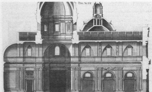
Fig. 29. Andrea Pozzo. "Perspectiva...", Sección de Sant' Ignazio de Roma, con la cúpula de Orazio Grassi (Fig. 94).
