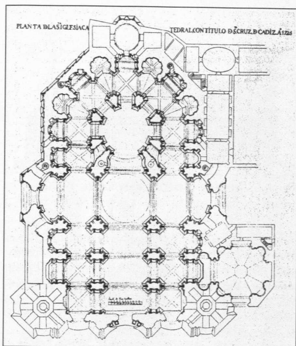
Fig. 5. Catedral de Cádiz. Planta de 1725 sobre el calco de Pablo Gutiérrez Moreno (1928).
