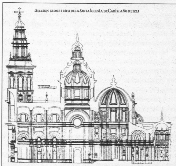
Fig. 7. Catedral de Cádiz. Sección longitudinal de 1725 sobre el calco de Pablo Gutiérrez Moreno (1928).
